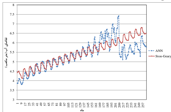
شکل ۵- مقایسه تقاضای سرانه آب پیش‌بینی شده با مدل استون‌گیری و شبکه عصبی برای دوره‌ی ۱۳۹۰-۱۴۱۰
