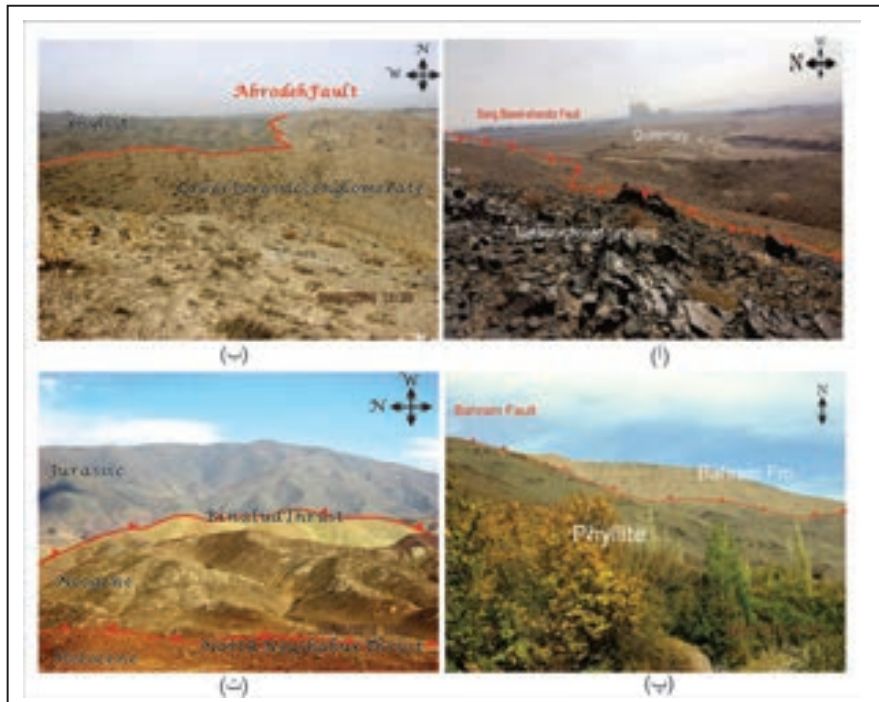
شکل ۲- آ) راندگی واحد پرمین (افیولیت مشهد) توسط گسل سنگ بست-شانددیز با شیب تقریبی ۵۰ درجه؛ ب) راندگی سنگ جوش ژوراسیک زیرین بر روی فیلیت مشهد شیب ۵۰ درجه؛ پ) راندگی سازند آهکی بهرام بر روی فیلیت‌های مشهد با شیب ۳۰ درجه؛ ت) راندگی واحدهای سنگی پالئوزوئیک بر روی سنگ‌های سنوزوئیک از طریق گسل بینالود با زاویه ۴۵ درجه شیب به سوی شمال خاور و در پایین عکس گسله شمال نیشابور با شیب ۶۰ درجه سنگ‌های آواری دوران سوم را بر روی نهشته‌های کواترنری قرار داده است.
