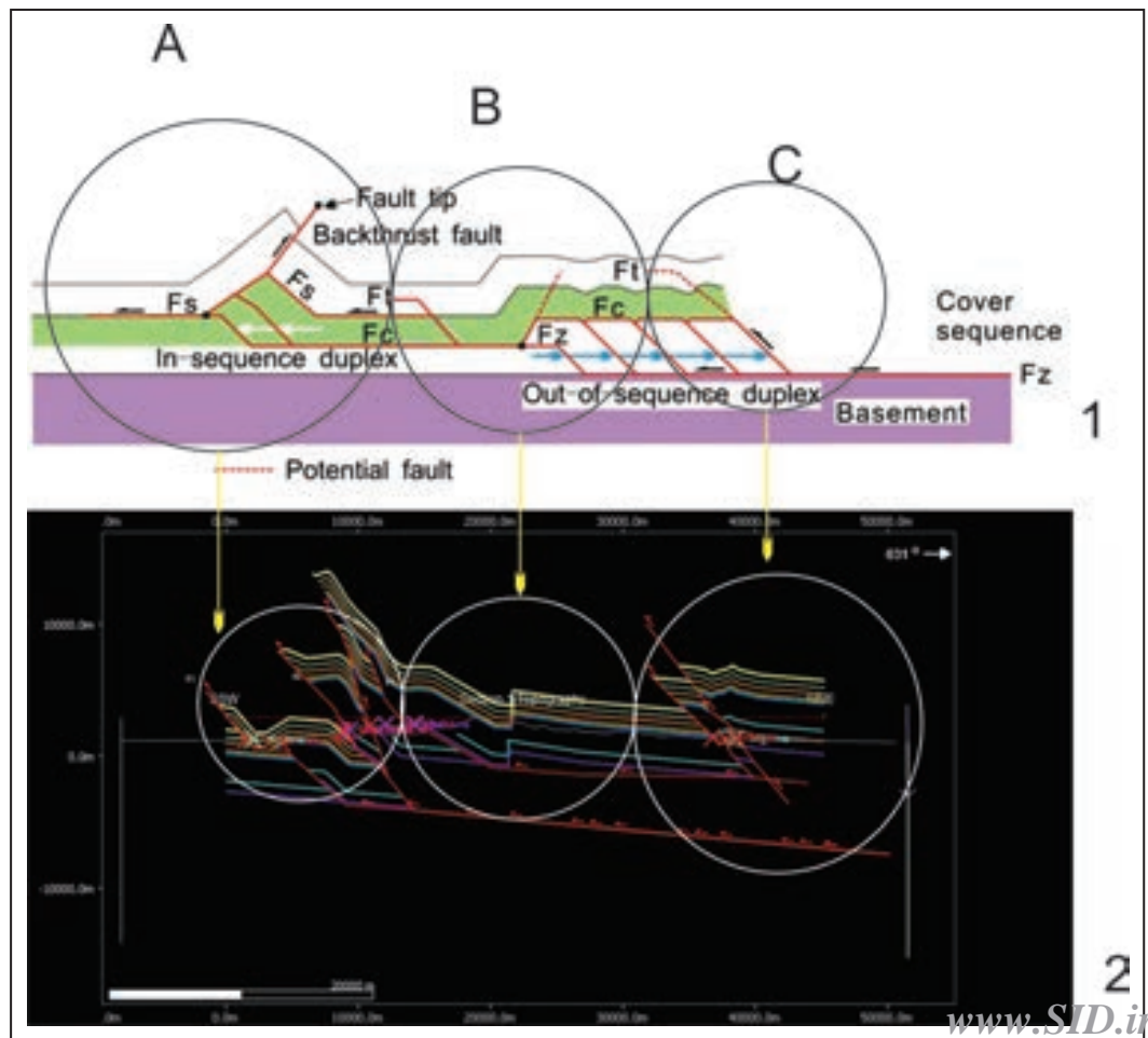
شکل ۶- مقایسه برش عرضی ترازمند شده گستره بینالود با مدل ساختاری گسله‌های بیرون از توالی برش عرضی ساختاری در چین که توسط Yan et al. (2009) ارائه شده است؛ (ب) برش عرضی ترازمند شده در گستره بینالود به کمک نرم‌افزار موو.
